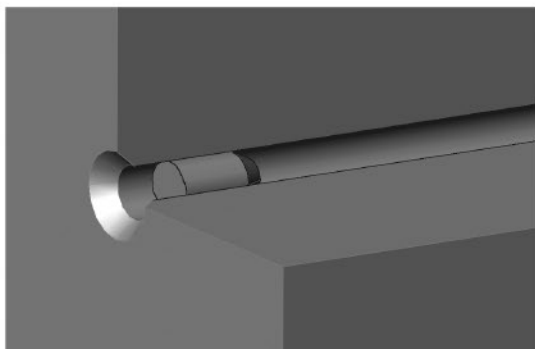
Rys. 4. Montaż korka Swell Sil w rurce dystansowej do ściągą
